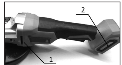
1. Εξαιρισμός Σχ. 17 2. Αεραγωγός εισαγωγής
